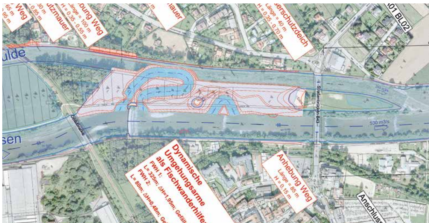
Planausschnitt - Hochwasserschutz Bauabschnitt 02.
